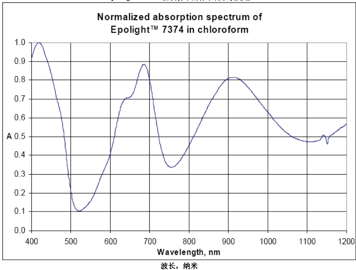
Epilight™ 7374 在氯仿中的标准化吸收光谱
