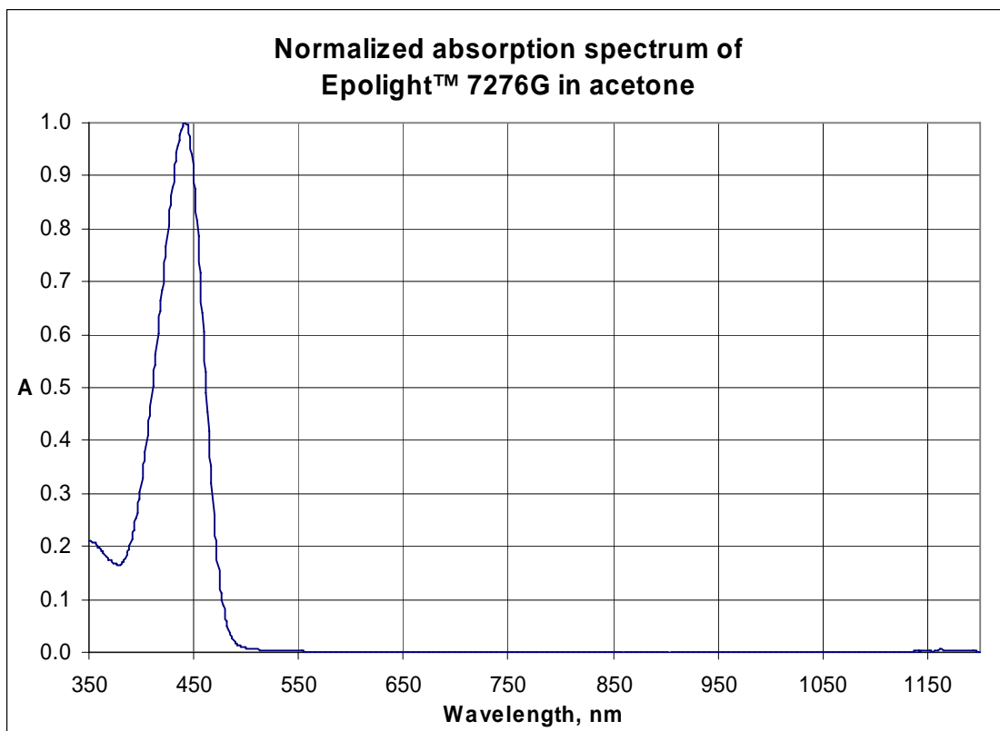
Epolight™ 7276G 在丙酮中的标准化吸收光谱
