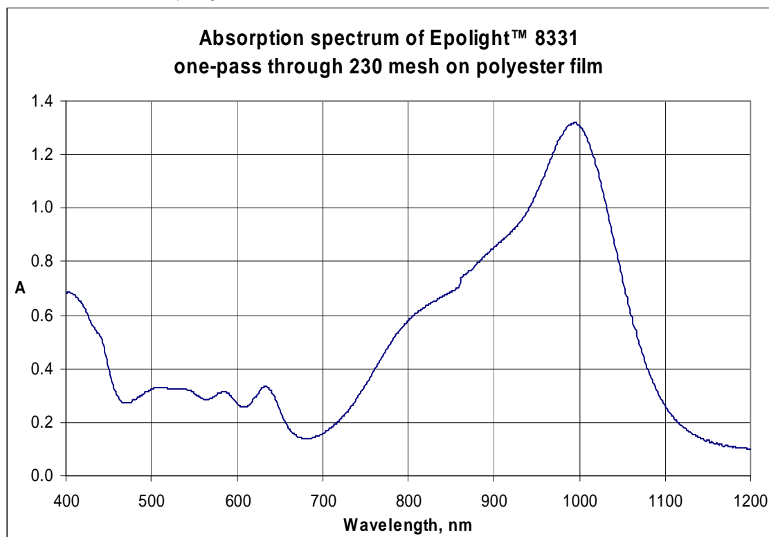
Epilight™ 8331 在聚酯薄膜上一次通过 230 目丝网的吸收图谱
