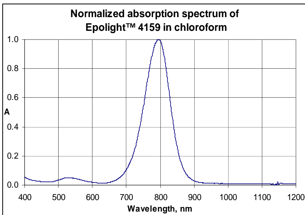
Epilight™ 4159 在氯仿中的标准化吸收光谱
