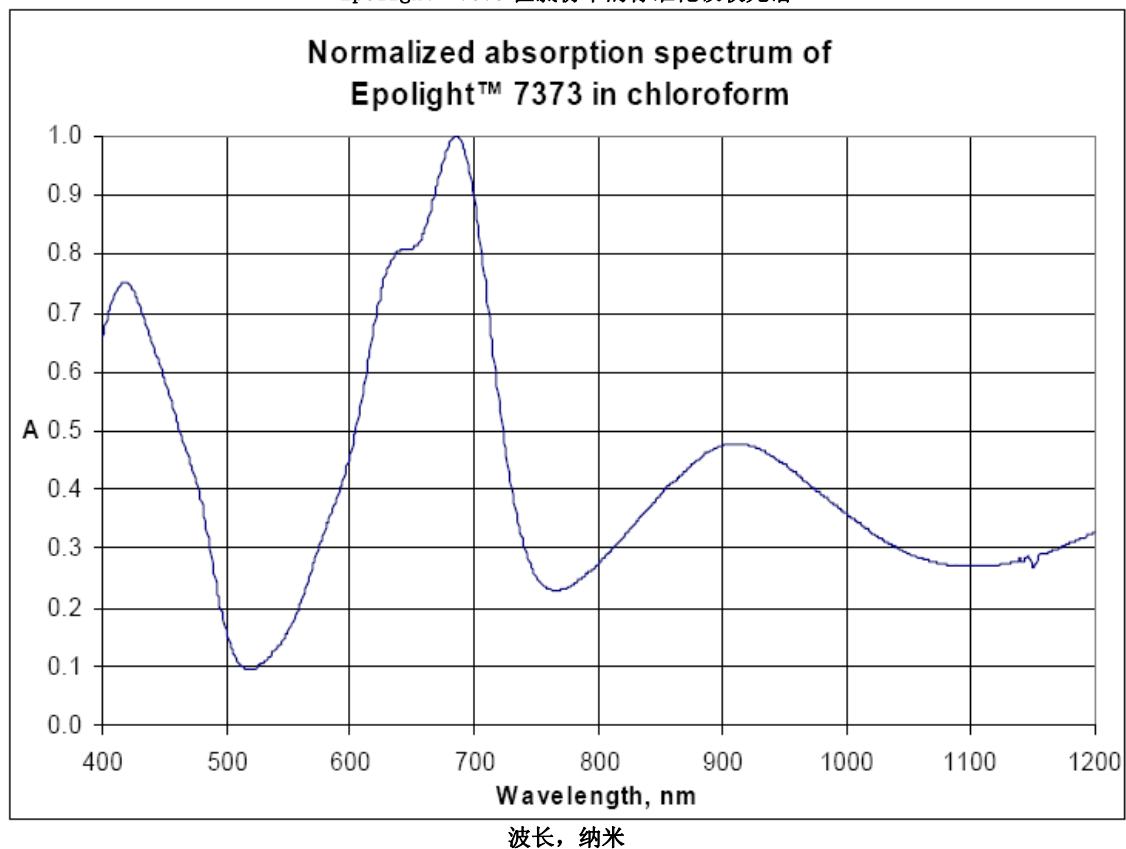
Epilight™ 7373 在氯仿中的标准化吸收光谱
