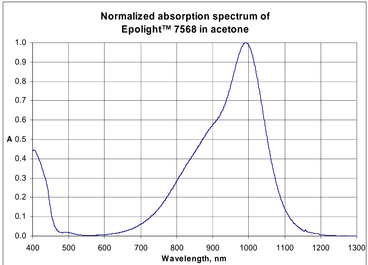
Epilight™ 7568 在丙酮中的标准化吸收光谱
