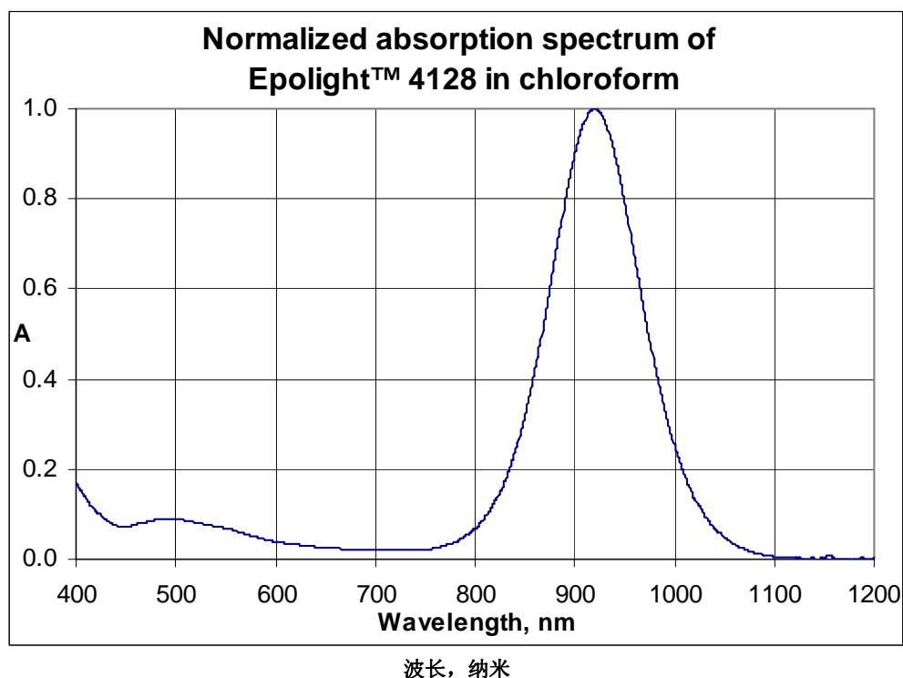
Epilight™ 4128 在氯仿中的标准化吸收光谱
