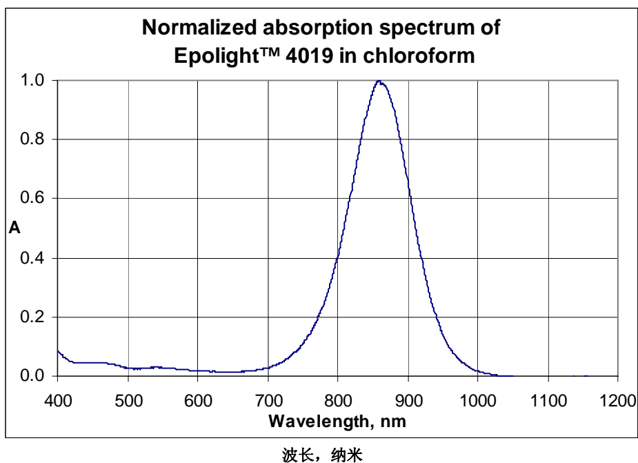
Epilight™ 4019 在氯仿中的标准化吸收光谱
