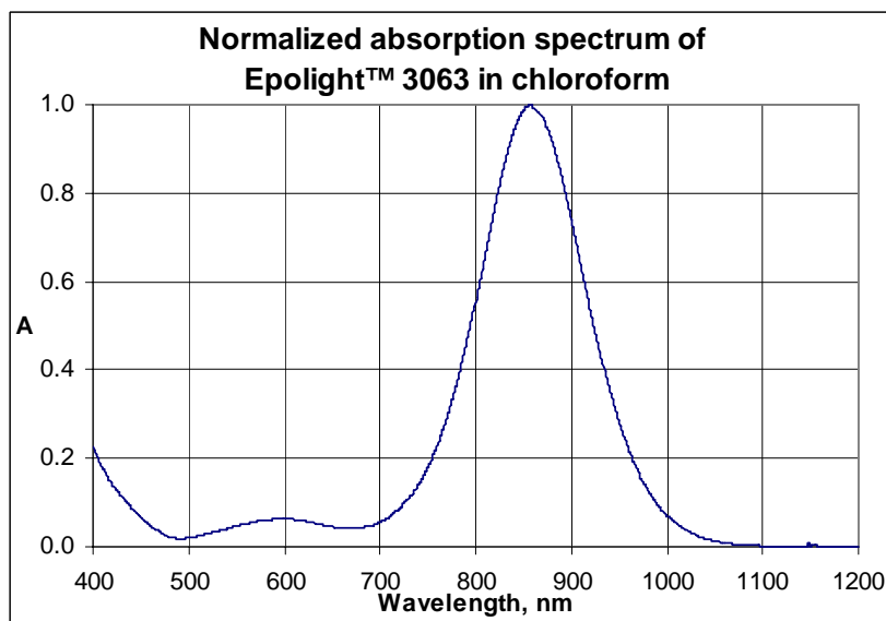
Epilight™ 3063 在氯仿中的标准化吸收光谱
