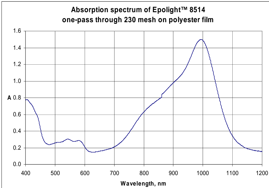
Epilight™ 8514 在聚酯薄膜上一次通过 230 目丝网的吸收图谱
