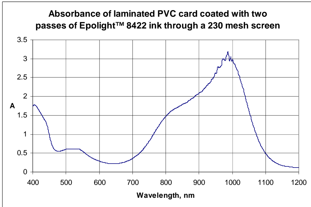
Epilight™ 8422 二次通过 230 目丝网层压 PVC 卡上的吸收图谱
