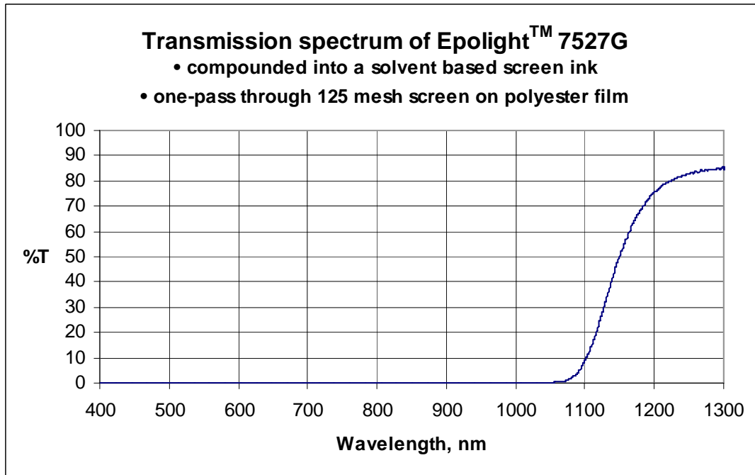
Epilight™ 7527G 透射光谱 (跟溶剂型丝印油墨混合，在聚酯薄膜上一次通过 125 目筛网)
