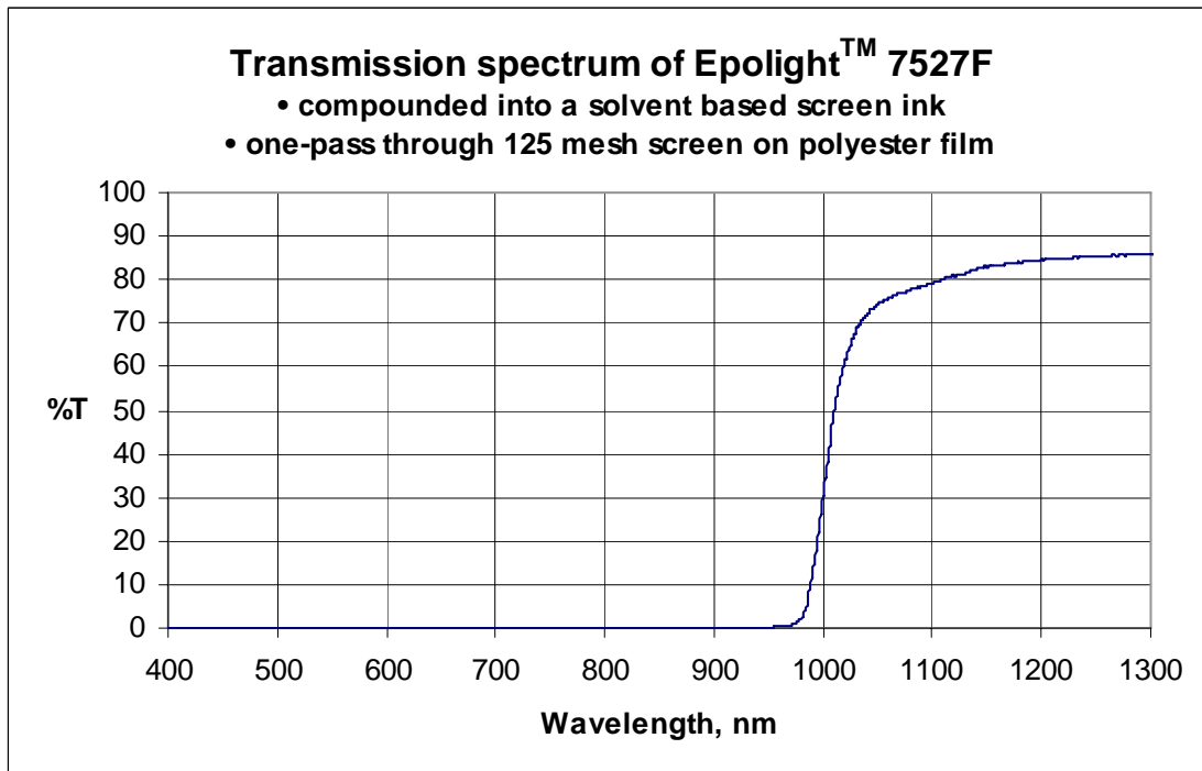
Epilight™ 7527F 透射光谱 (跟溶剂型丝印油墨混合, 在聚酯薄膜上一次通过 125 目筛网)
