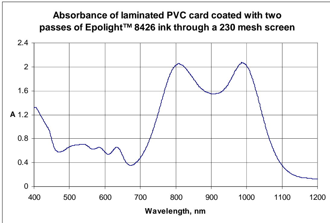
Epilight™ 8426 二次通过 230 目丝网层压 PVC 卡上的吸收图谱
