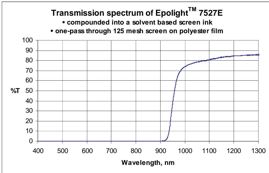
Epilight™ 7527E 透射光谱 (跟溶剂型丝印油墨混合, 在聚酯薄膜上一次通过 125 目筛网)
