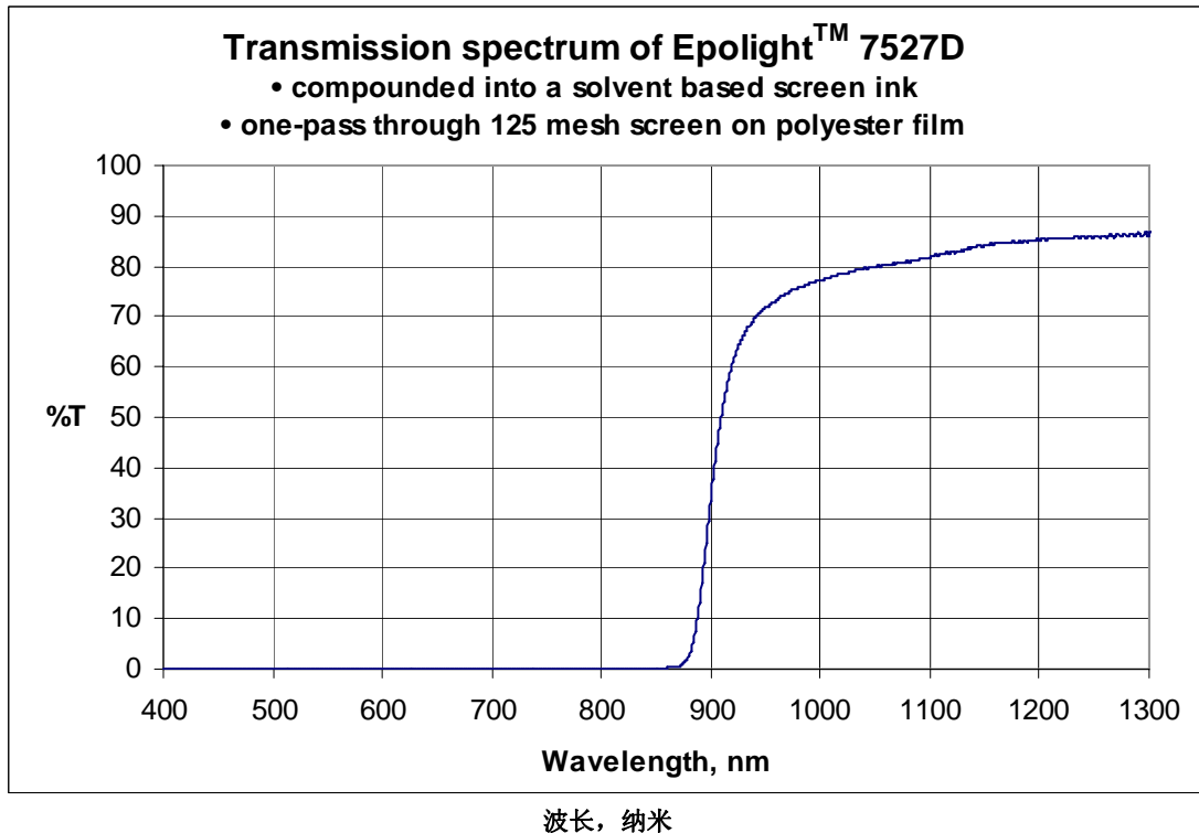
Epilight™ 7527D 透射光谱 (与溶剂型丝印油墨混合, 在聚酯薄膜上一次通过 125 目筛网)
