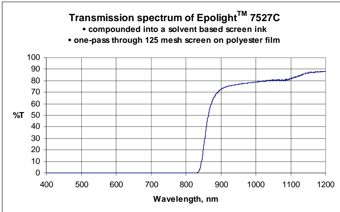
Epilight™ 7527C 透过率光谱 (与溶剂型丝印油墨混合，在聚酯薄膜上一次通过 125 目筛网)
