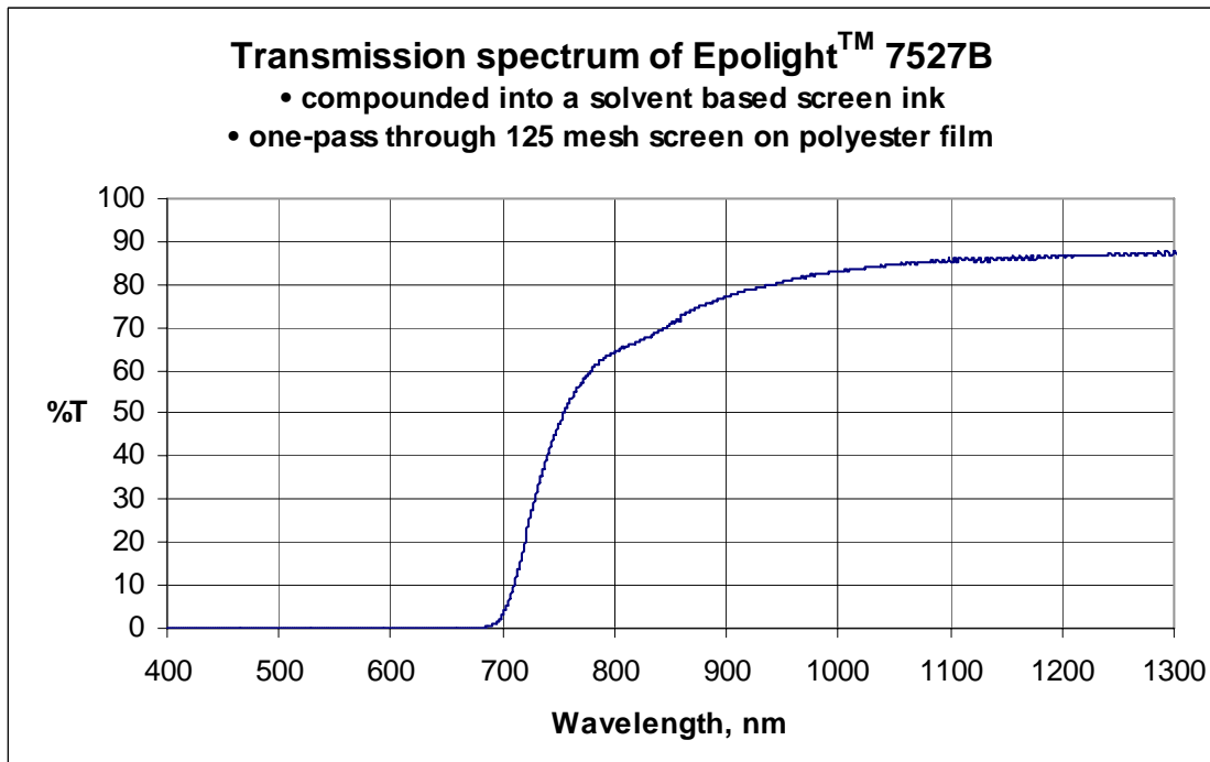
Epilight™ 7527B 透射光谱 (与溶剂型丝印油墨混合, 在聚酯薄膜上一次通过 125 目筛网)
