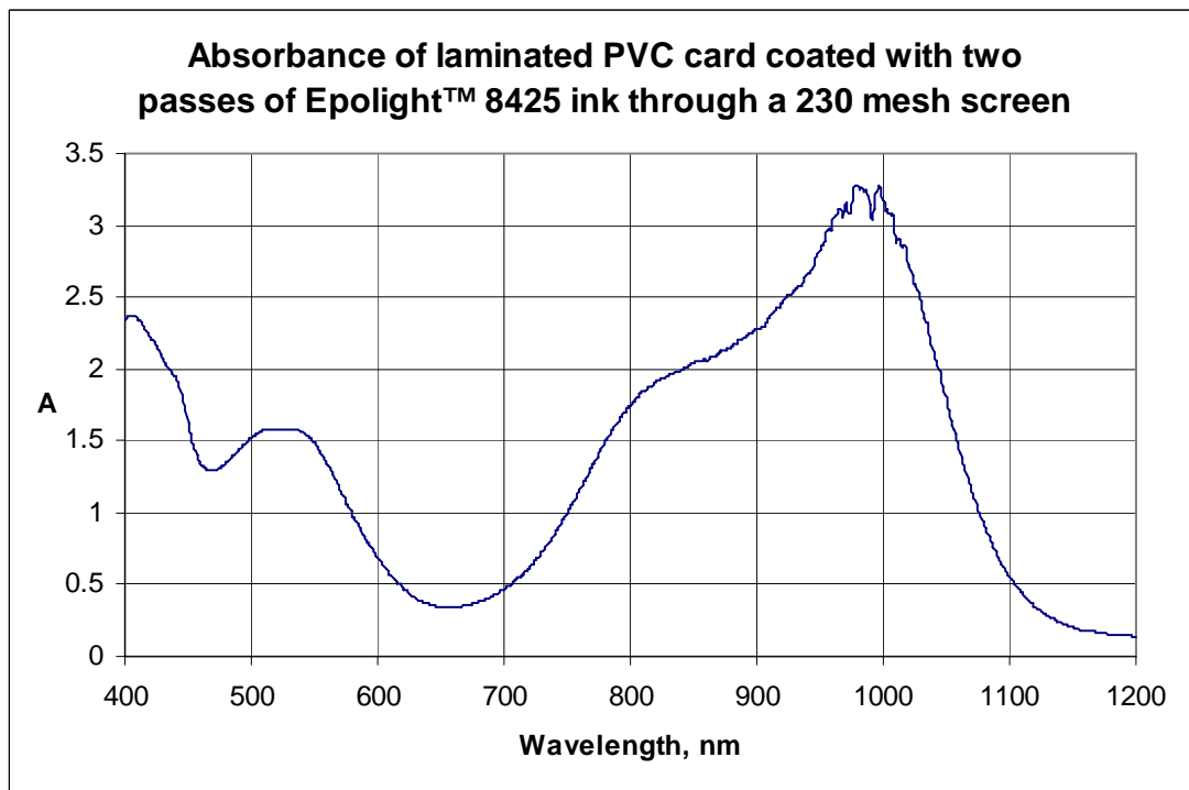
Epolight™ 8425 二次通过 230 目丝网层压 PVC 卡上的吸收图谱
