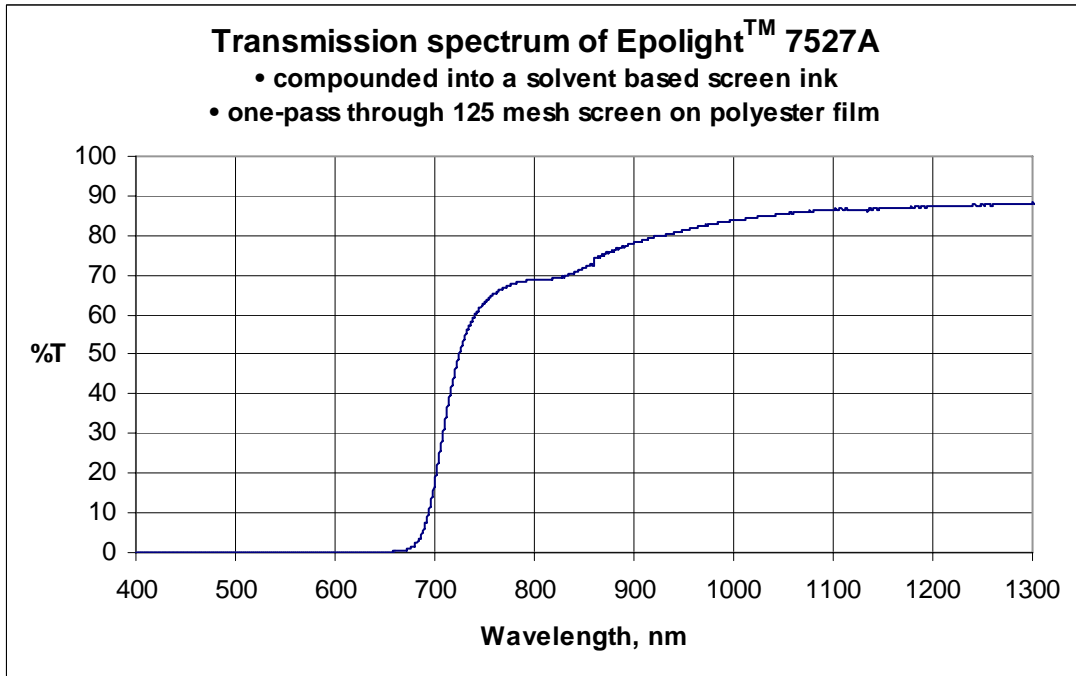
Epilight™ 7527A 透过光谱 (与溶剂型丝印油墨混合, 在聚酯薄膜上一次通过 125 目筛网)
