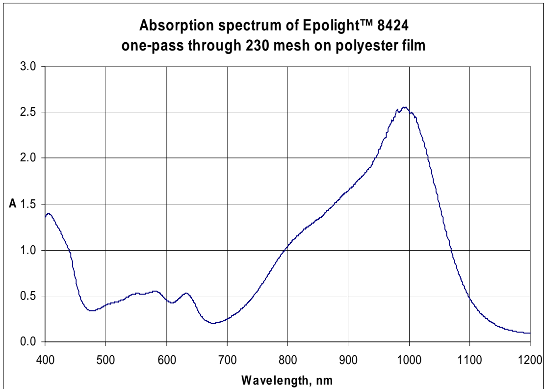
Epolight™ 8424 在聚酯薄膜上一次通过 230 目丝网的吸收图谱
