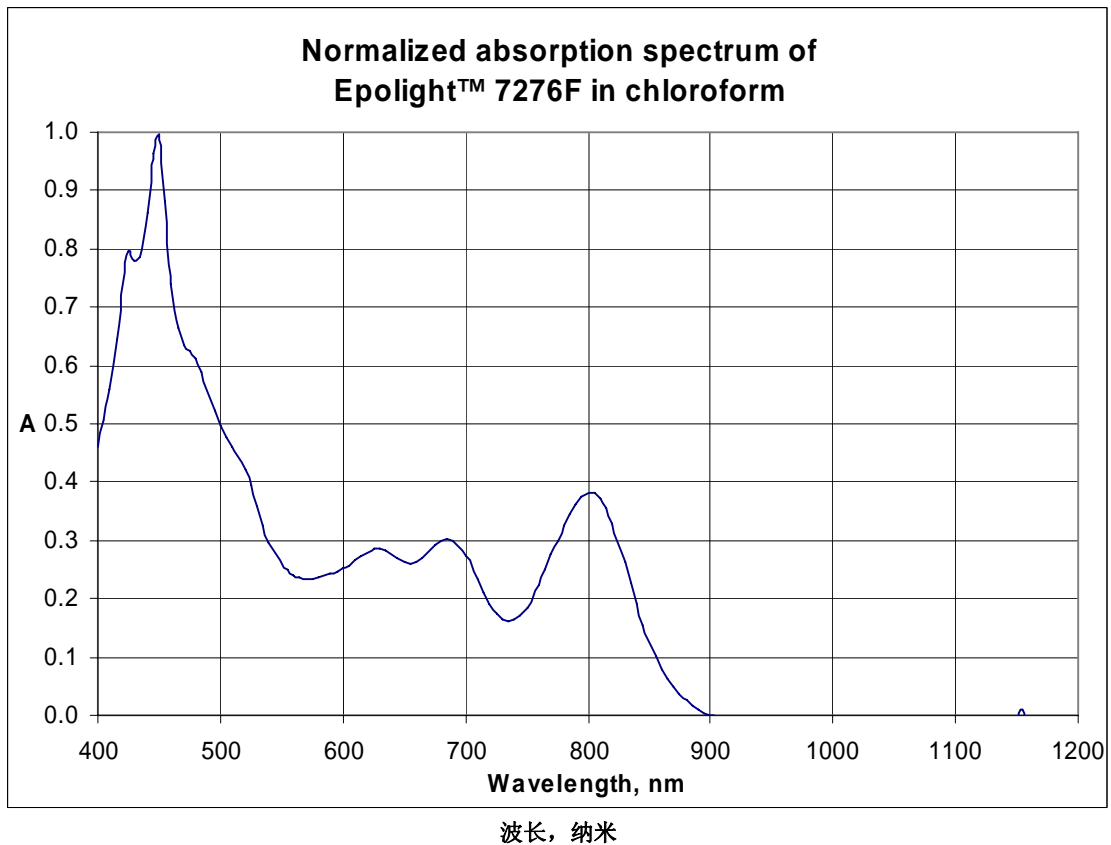
Epolight™ 7276F 在氯仿中的标准化吸收光谱
