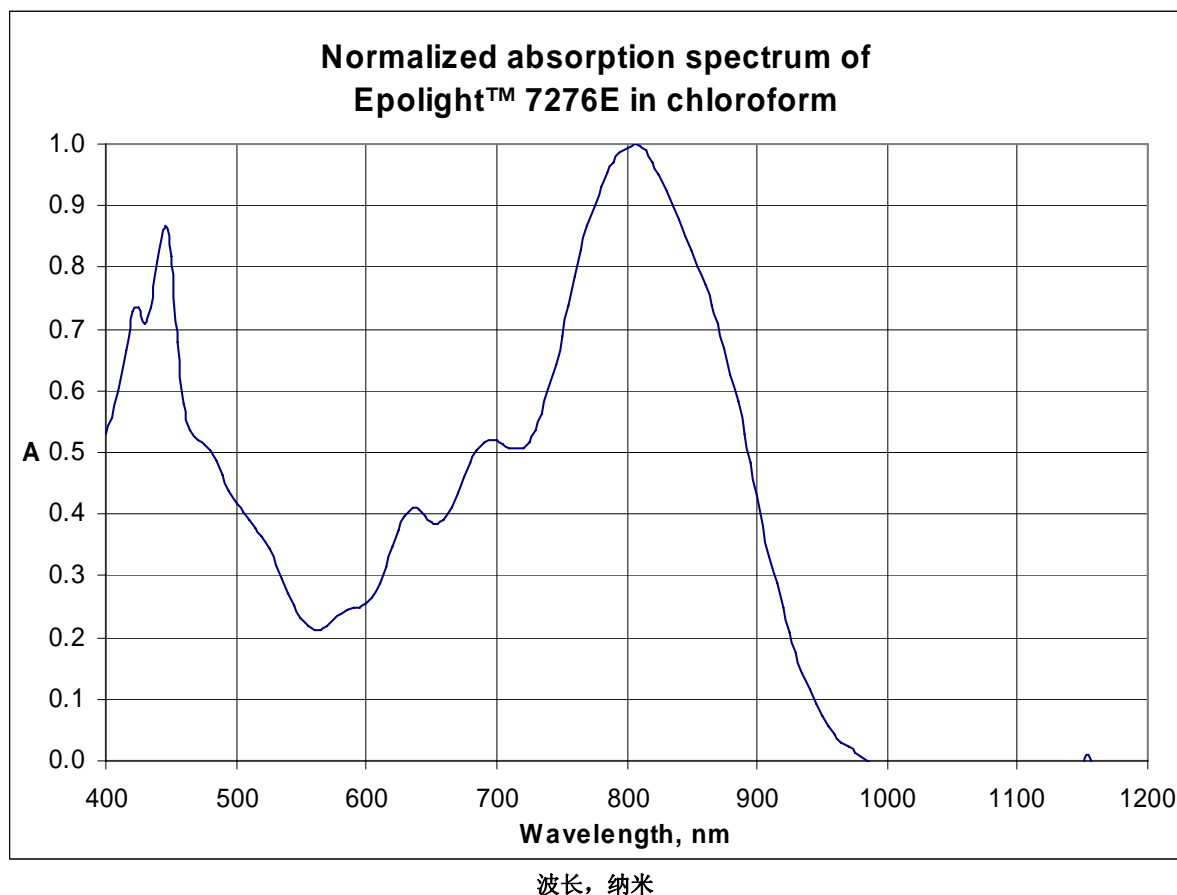
Epilight™ 7276E 在氯仿中的标准化吸收光谱
