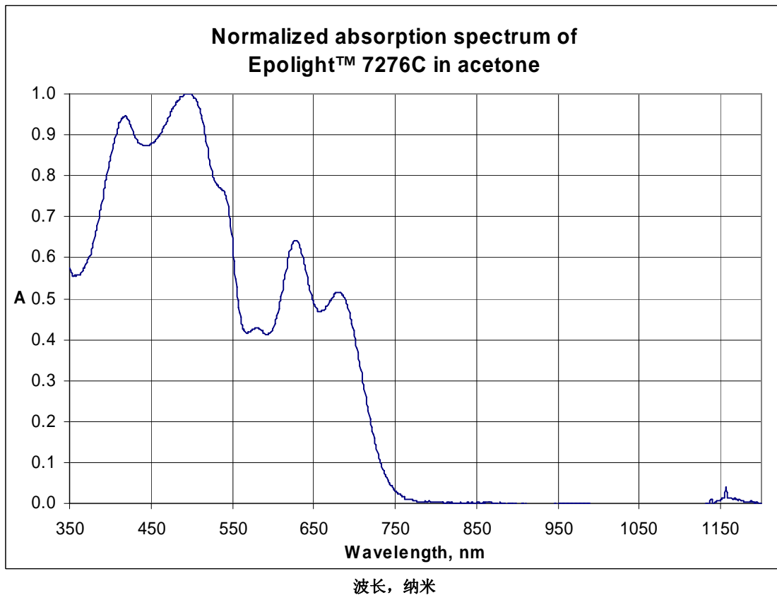
Epolight™ 7276C 在丙酮中的标准化吸收光谱
