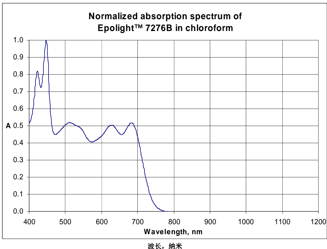
Epolight™ 7276B 在氯仿中的标准化吸收光谱
