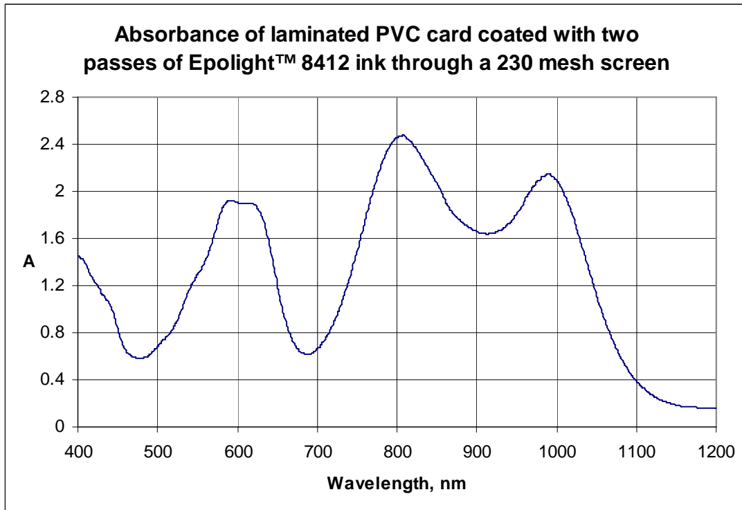
Epilight™ 8412 二次通过 230 目丝网在层压 PVC 卡上的吸收图谱
