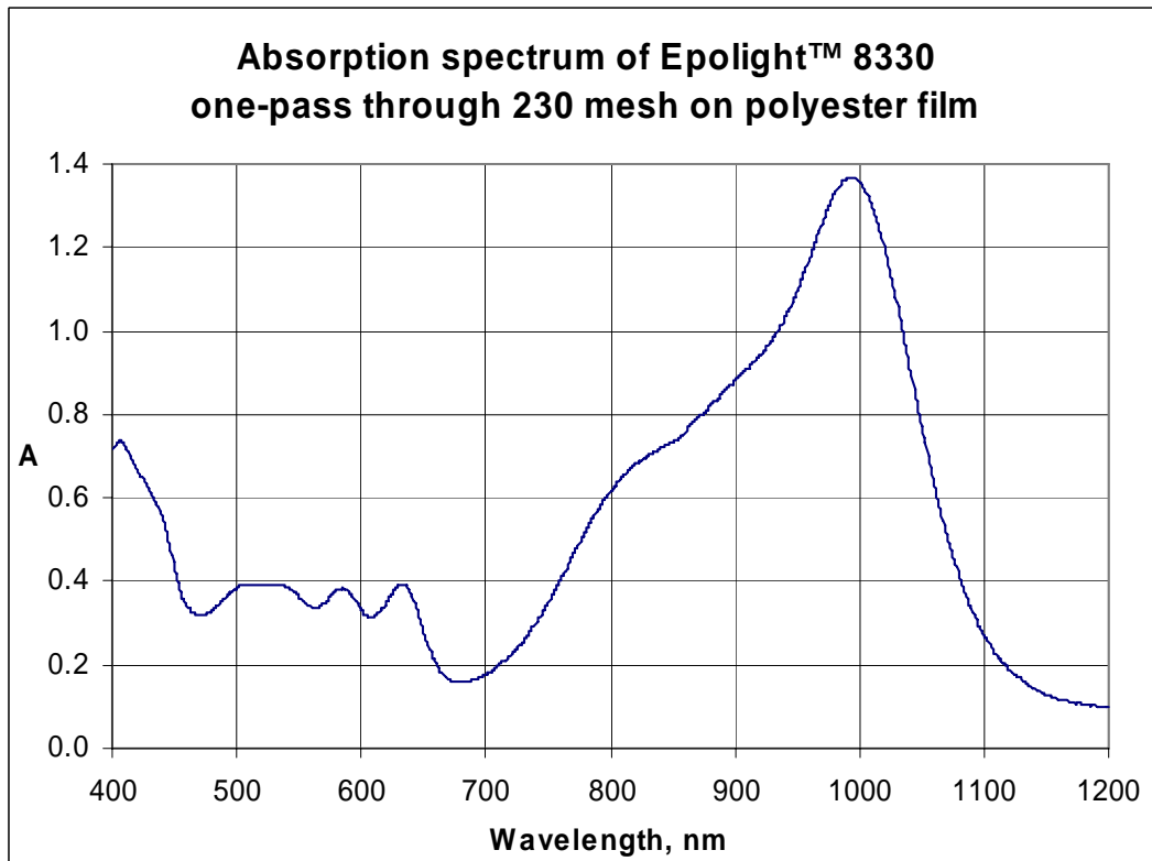
Epilight™ 8330 在聚酯薄膜上一次通过 230 目丝网的吸收图谱
