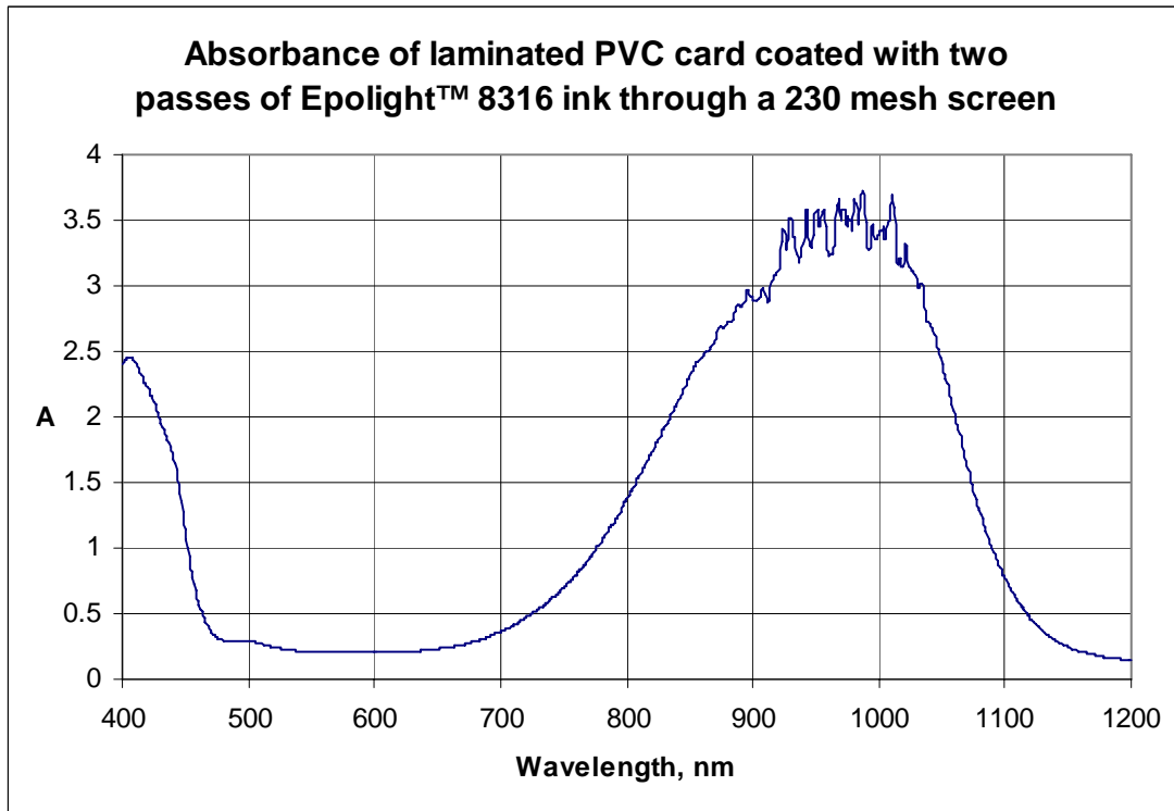
Epilight™ 8316 油墨以两次通过 230 目丝网涂覆的层压 PVC 卡之吸收图谱
