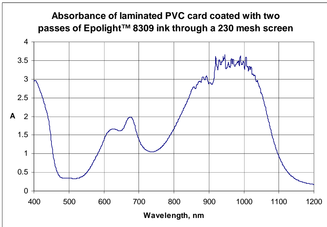
Epilight™ 8309 油墨以两次通过 230 目丝网涂覆的层压 PVC 卡之吸收图谱
