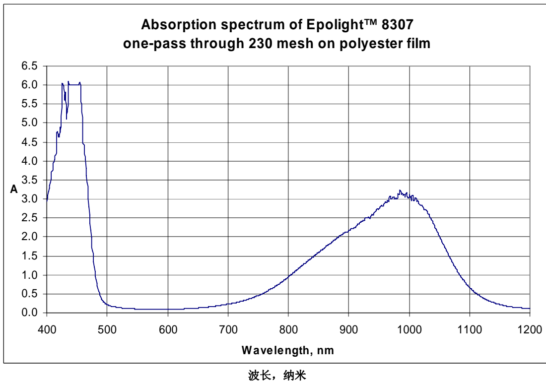
Epilight™ 8307 在聚酯薄膜上一次通过 230 目筛的吸收光谱
