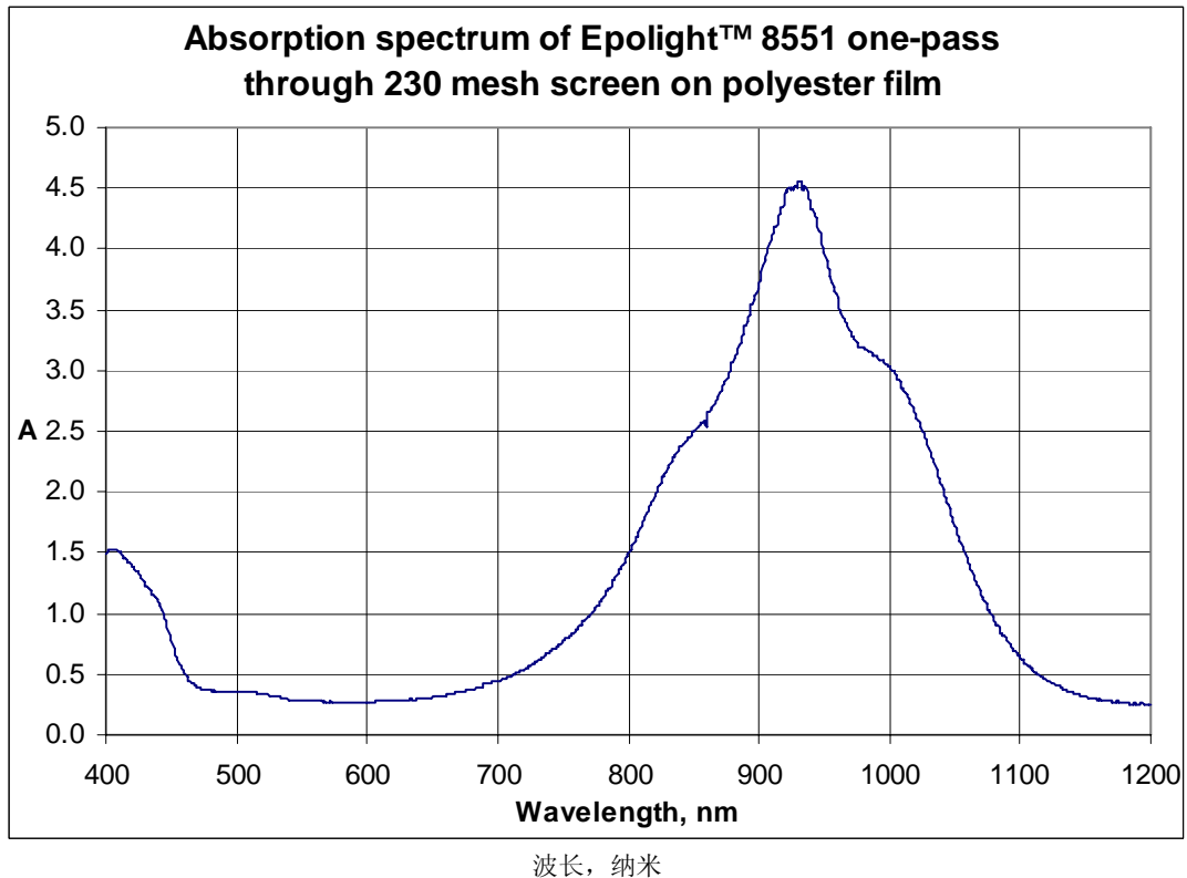
Epilight™ 8551 在聚酯薄膜上一次通过 230 目丝网的吸收图谱
