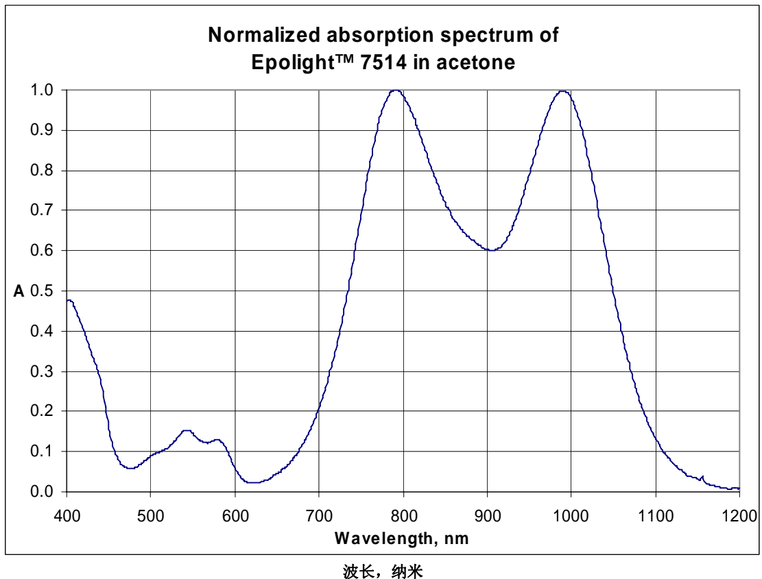
Epilight™ 7514 在丙酮中的标准化吸收光谱
