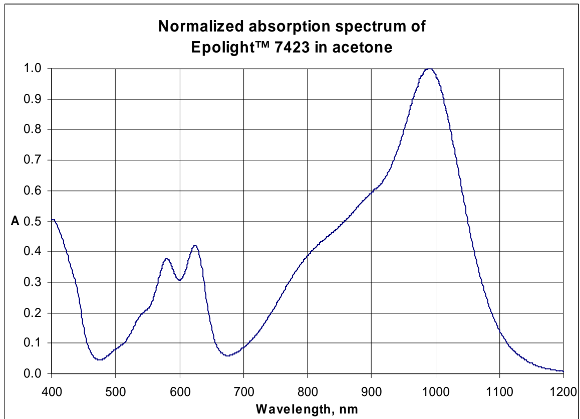
Epilight™ 7423 在丙酮中的标准化吸收光谱
