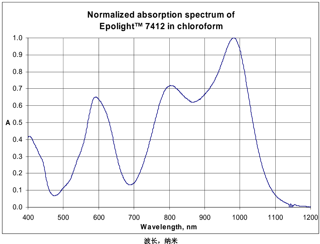
Epilight™ 7412 在氯仿中的标准化吸收光谱
