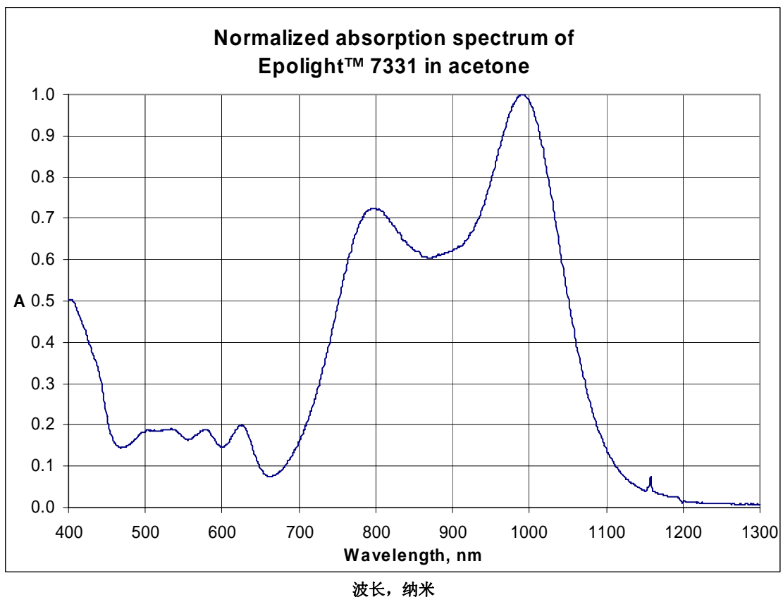
Epilight™ 7331 在丙酮中的标准化吸收光谱
