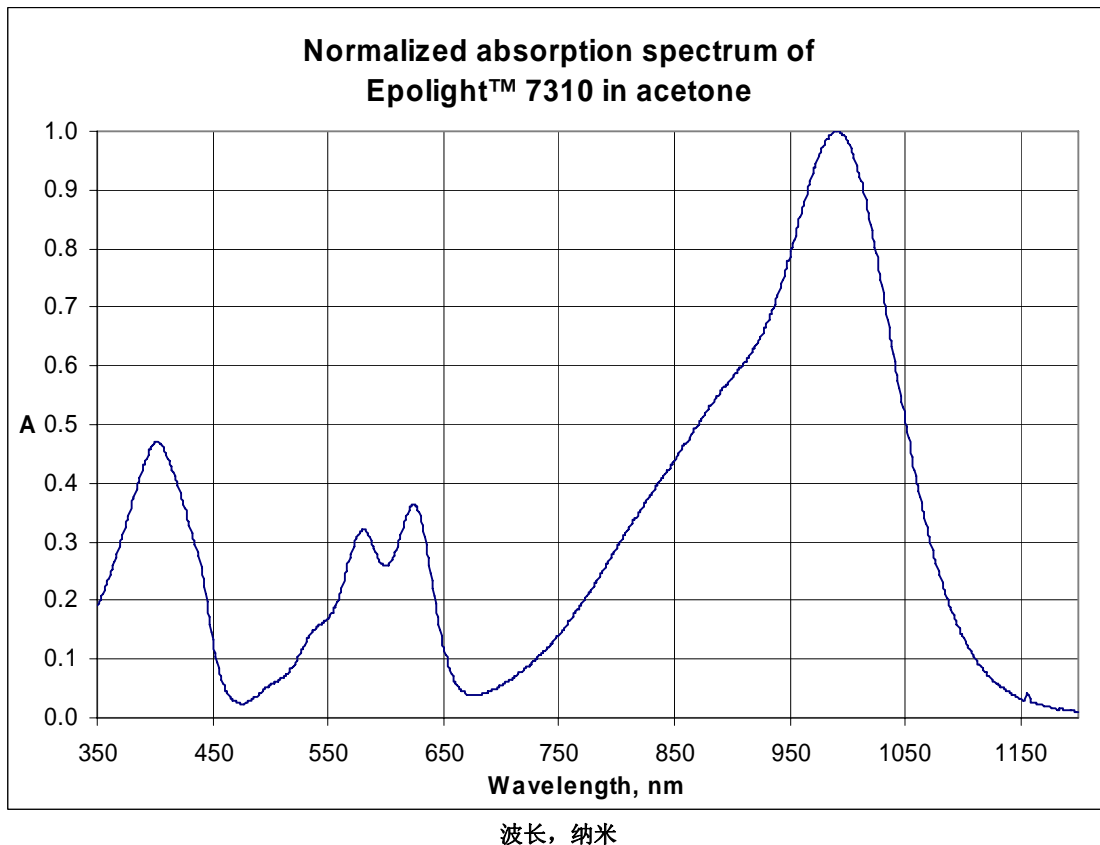
Epilight™ 7310 在丙酮中的标准化吸收光谱
