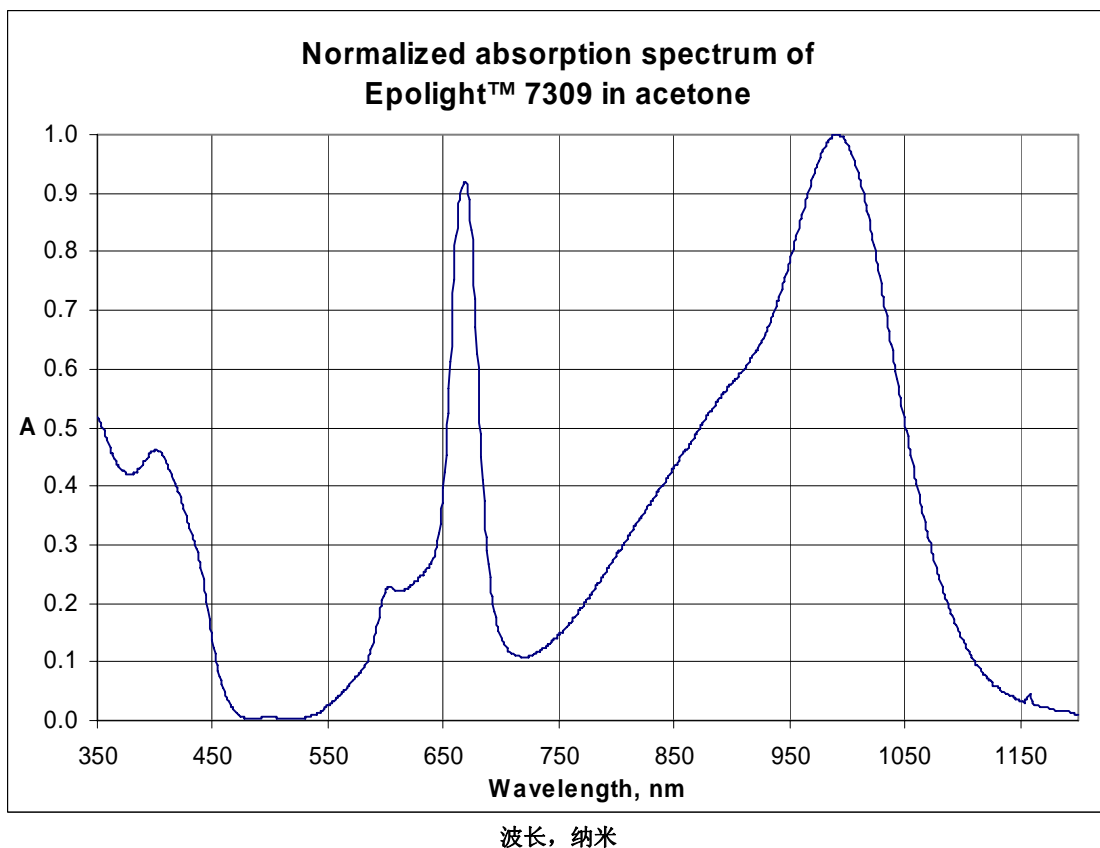
Epilight™ 7309 在丙酮中的标准化吸收光谱
