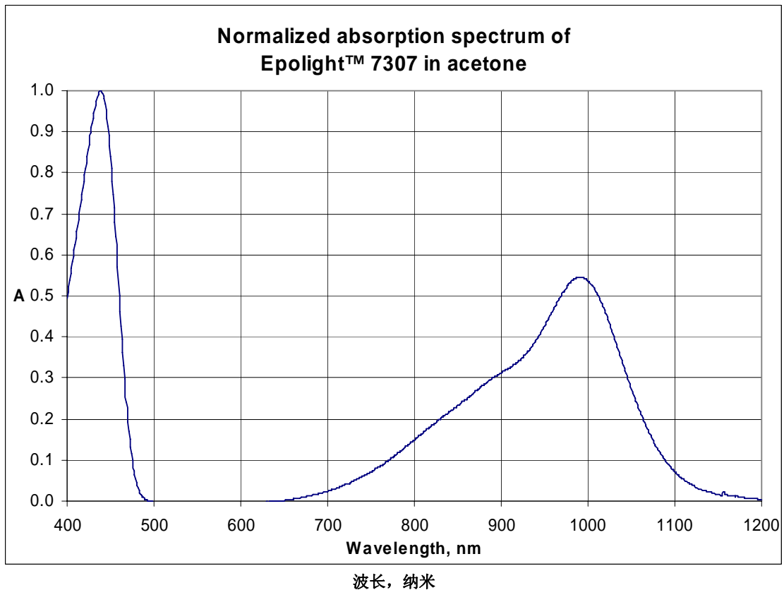
Epilight™ 7307 在丙酮中的标准化吸收光谱
